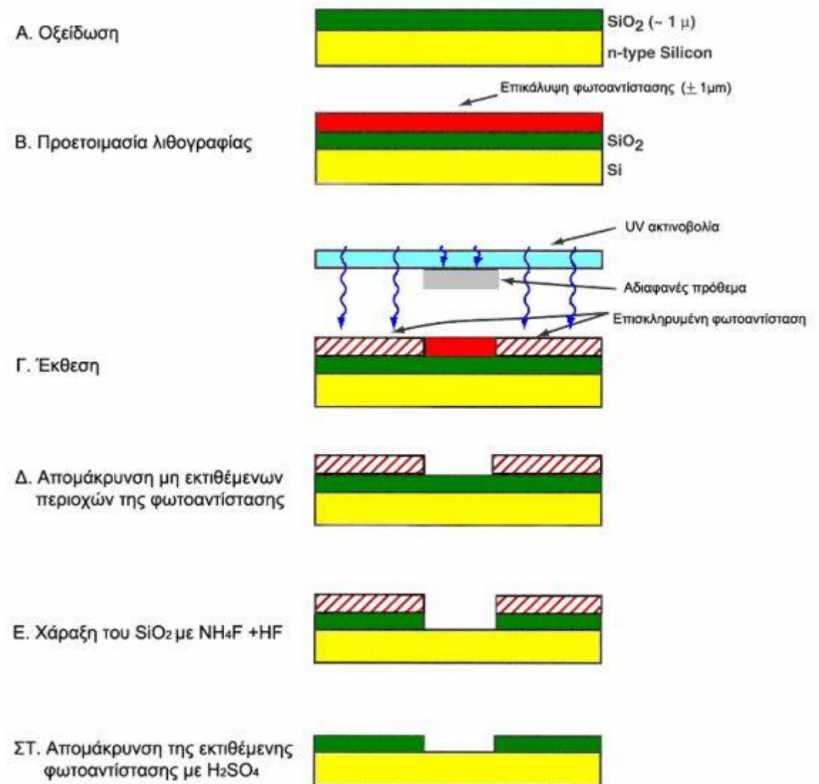
Σχήμα 2.1 Διαδοχικές φάσεις της φωτολιθογραφίας
